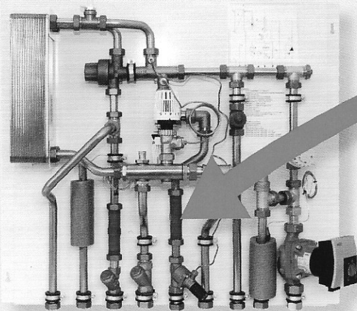
Frischwarmwasserstation
